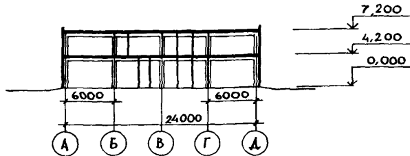
РАЗРЕЗ I-I
