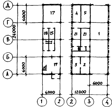
ПЛАН НА ОТМ. 4.200
