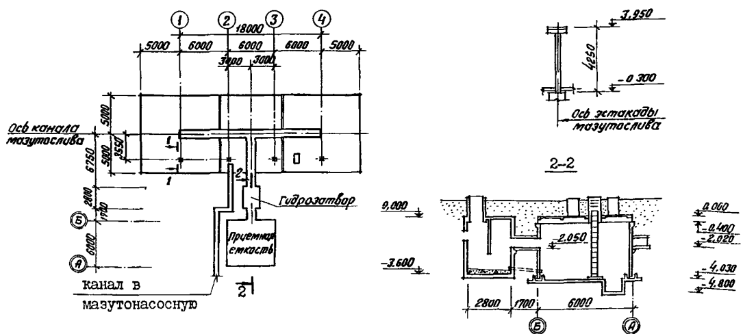
СООРУЖЕНИЯ СЛИВА И ПРИЕМА МАЗУТА
