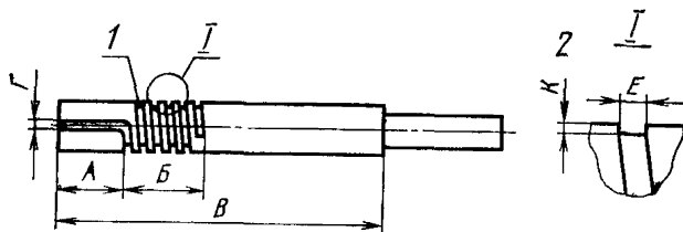
1—винтовая канавка; 2—канавка в увеличенном виде
