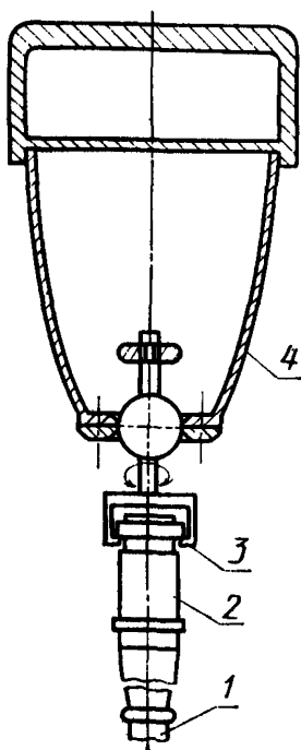
1—кабель; 2—разъем; 3—подшипник; 4—захват
