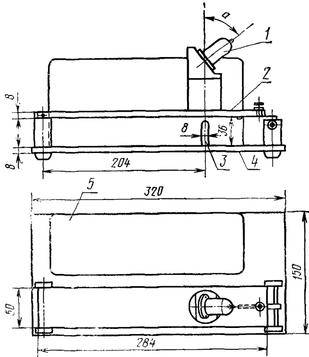
1—испытуемая лампа; 2—падающая платформа; 3—наковальня; 4—основание; 5—кожух, содержащий элементы схемы
