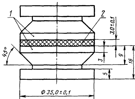
1 — металлические диски; 2 — резина
