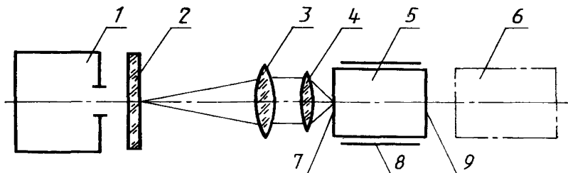
1—осветитель; 2—сетка; 3—коллимационный объектив; 4—проекционный объектив; 5—ЭОП; 6—яркомер; 7—фотокатод; 8—светонепроницаемая камера; 9—экран
