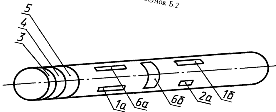
D_n св. 60 до 120 мм Рисунок Б.3
