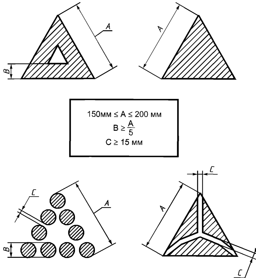
Рисунок 1 — Отражатели света для прицепов класса III A
