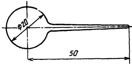
Рисунок 1 — Ампула стеклянная сферическая
