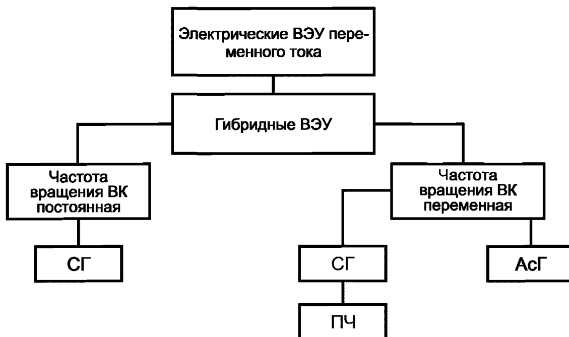
Рисунок 3 — Структурная схема системных ВЭУ
