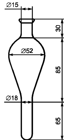
Рисунок 2 — Колба специальная для титрования
