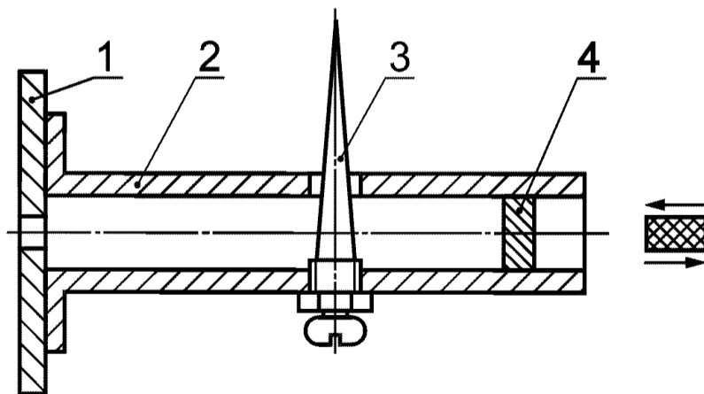
1 — диафрагма; 2 — волновод (10 × 23); 3 — антенна; 4 — поршень настройки
