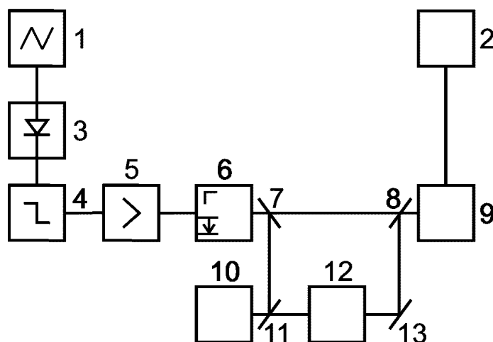
1 — осциллограф; 2 — испытуемое изделие; 3 — частотный детектор; 4 — ограничитель; 5 — полосовой усилитель на частоту 30 мГц; полоса пропускания 0,5 мГц; 6 — фотоприемник; 7, 8, 11 — полупрозрачное зеркало (с коэффициентом отражения не менее 50 %); 9 — фокусирующая система; 10 — газовый оптический квантовый генератор; 12 — устройство для сдвига частоты; 13 — зеркало с коэффициентом отражения не менее 90 %
