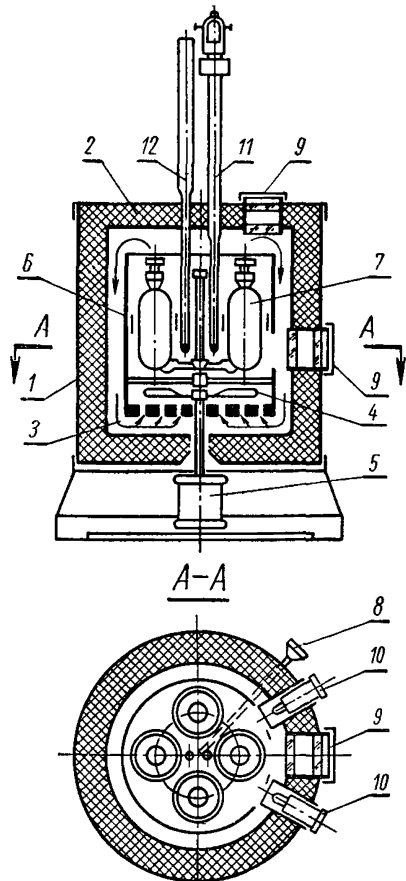
Схема прибора для окисления
