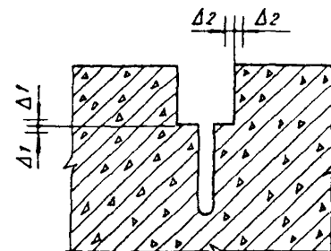
Схема поперечного разреза шва с указанием предельных отклонений
