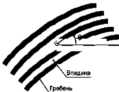
Рисунок 4 — Расположение контрольной точки окончания основы гребней
