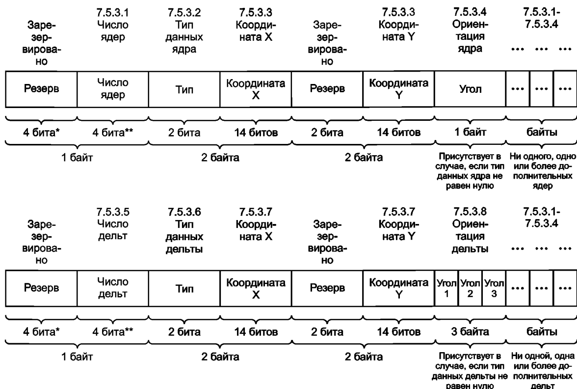
Рисунок 8 — Диаграмма формата данных ядра и дельты
