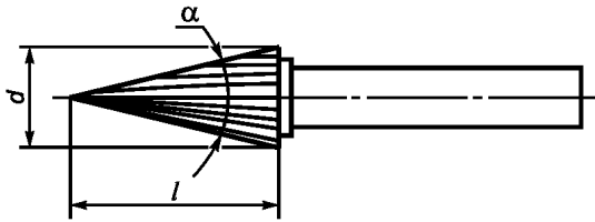
Рисунок 10 — Борфрезы типа М
