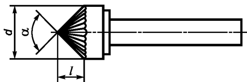
Рисунок 8 — Борфрезы типа J и K
