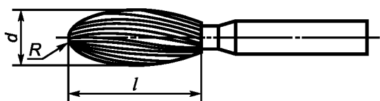
Рисунок 7 — Борфрезы типа H
