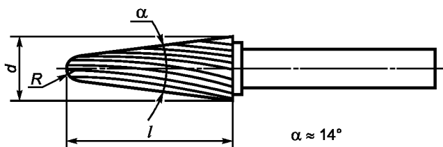
Рисунок 9 — Борфрезы типа L
