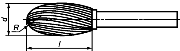
Рисунок 4 — Борфрезы типа E
