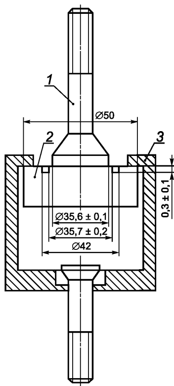
1 — испытательная головка; 2 — образец; 3 — захват
