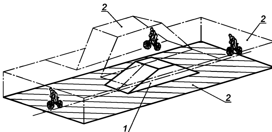
1 — оборудование; 2 — зона безопасности
