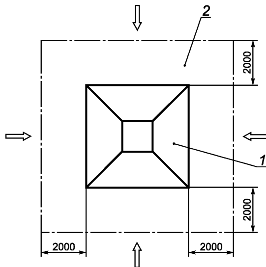
1 — пирамида; 2 — зона безопасности
