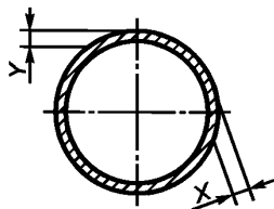
Рисунок 4 — Выступ ребра по краю поверхности катания
