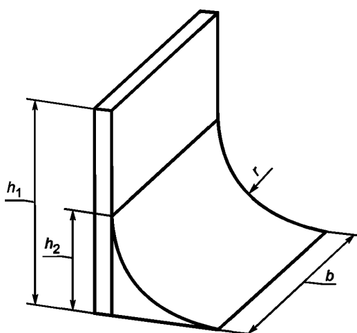
Рисунок 12 — Ramпа со стеной
