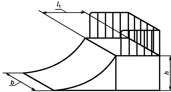
Рисунок 10 — Рампа для прыжков с платформой
