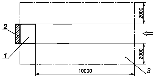
1 — рампа; 2 — стена; 3 — зона безопасности
