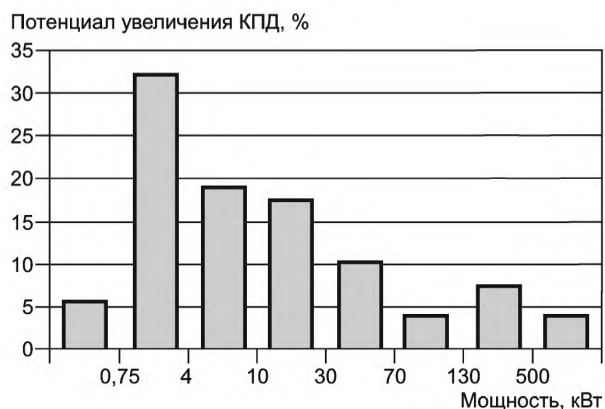
Рисунок 1 — Распределение потенциала энергосбережения двигателей по мощностям
