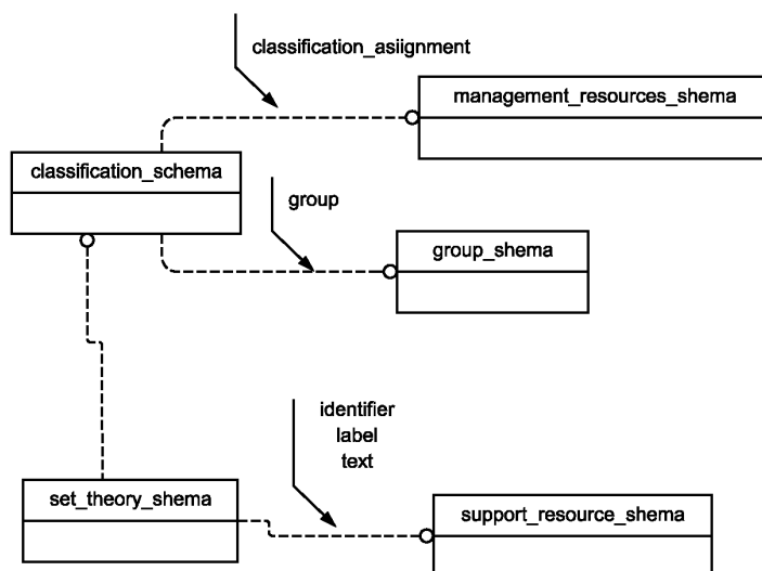
Рисунок 1 — Отношения между схемами по ИСО 10303-54
