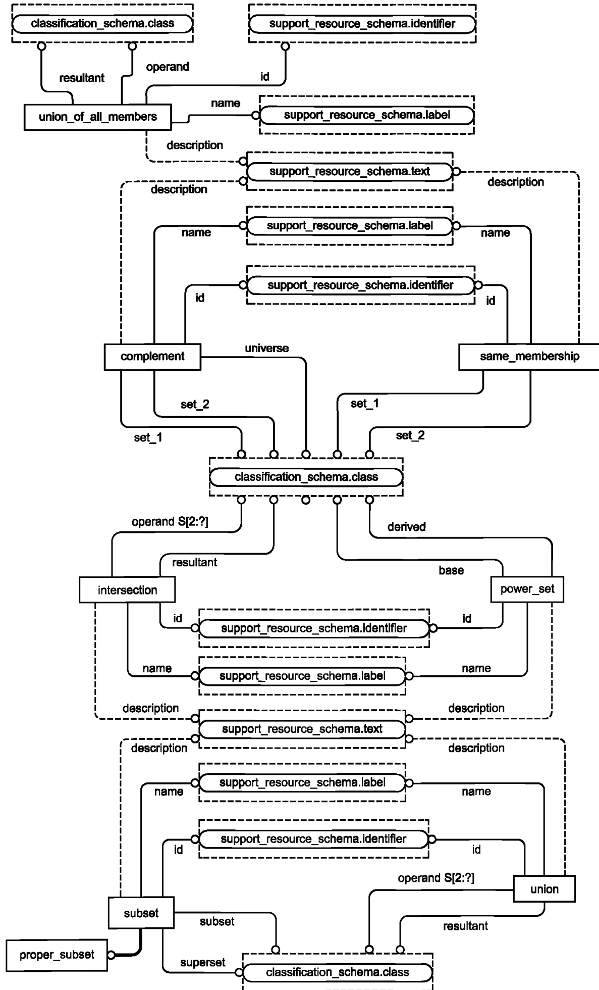
Рисунок D.2 — EXPRESS-G диаграмма схемы set_theory_schema
