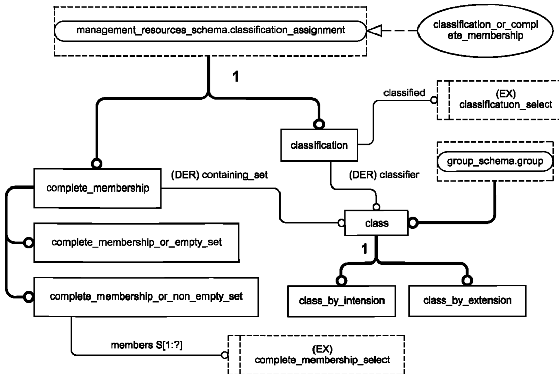
Рисунок D.1 — EXPRESS-G диаграмма схемы classification_schema
