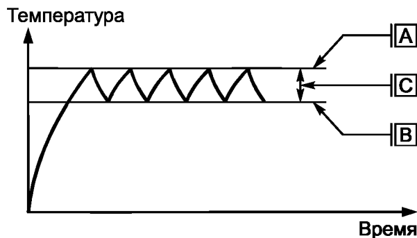
Рисунок EE.2 — Термоограничитель с самовозвратом
