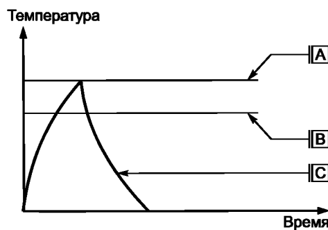
Рисунок EE.3 — Термоограничитель без самовозврата
