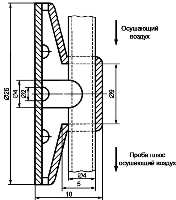
Рисунок 9 — Пробоотборник
