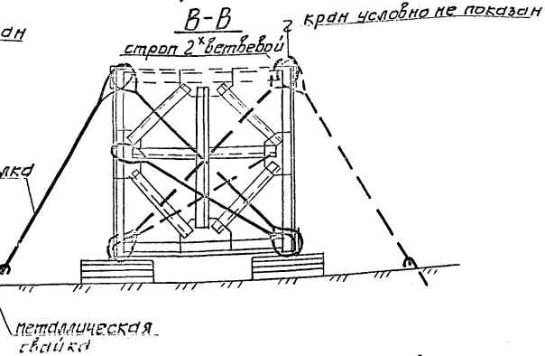
Рис. 1-3 Сборка анкерно-узловой опоры УСК 500-1
