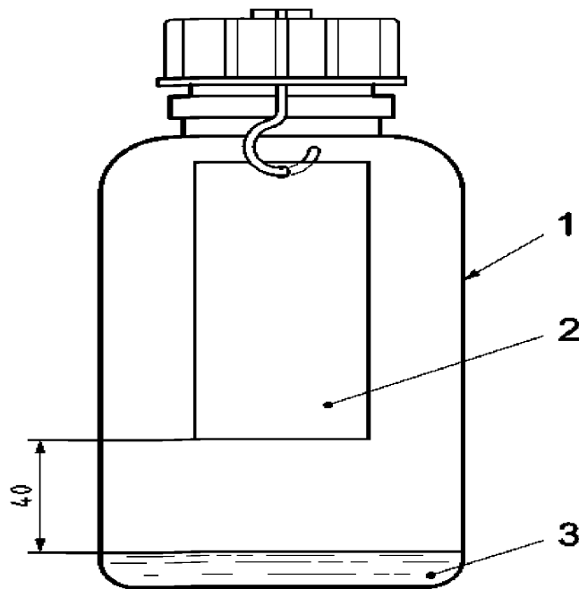
1 – сосуд из полиэтилена; 2 – образец; 3 – вода
