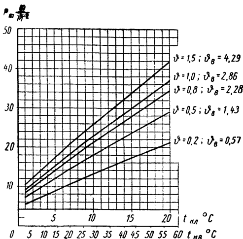
Рис. 1. График зависимости статического давления льда от температуры и градиента температуры льда \theta — градиент температуры льда; \theta_{в} — градиент температуры воздуха
