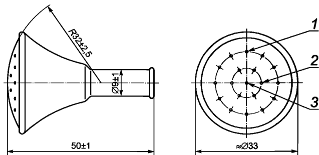
Рисунок 2 — Разбрызгивающее сопло
