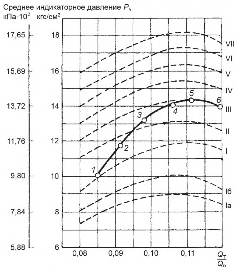
Рисунок 1 – Кривая детонационных характеристик
