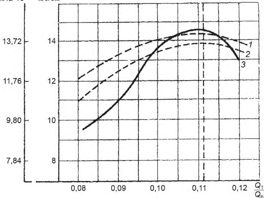
Рисунок 2 – Детонационная характеристика топлива
