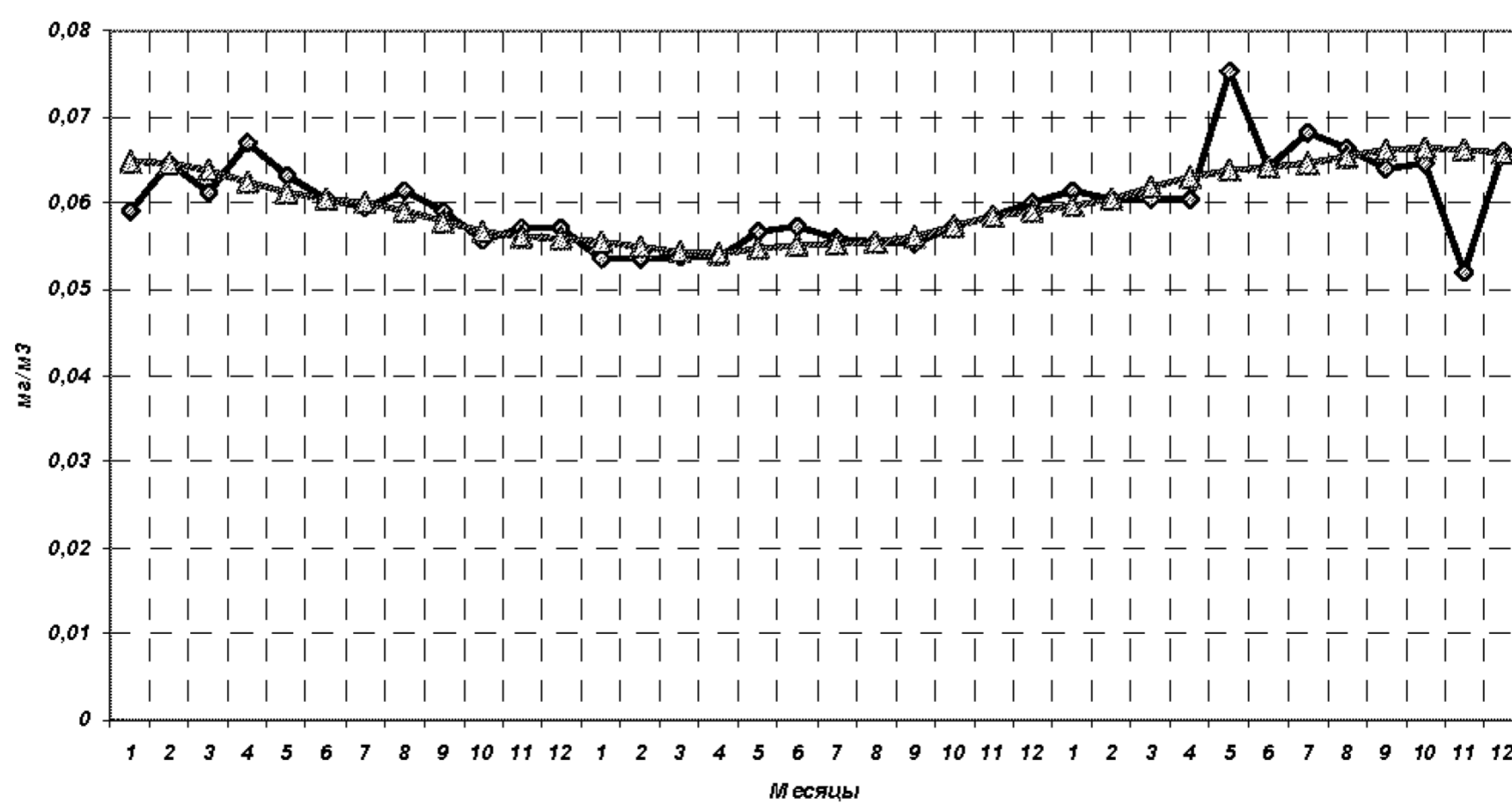
г) PM 10
