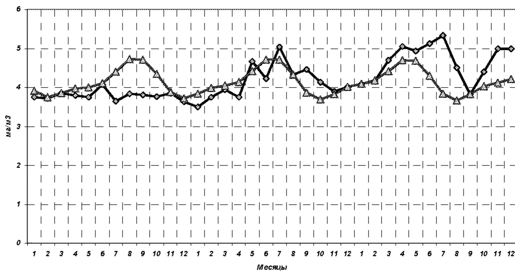
б) CO
