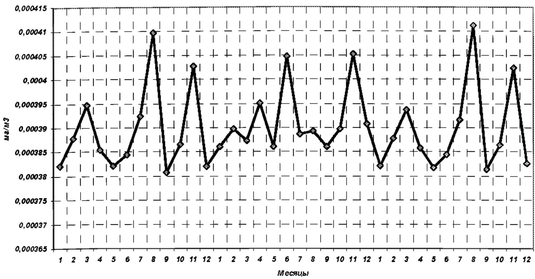
Д) Cd
