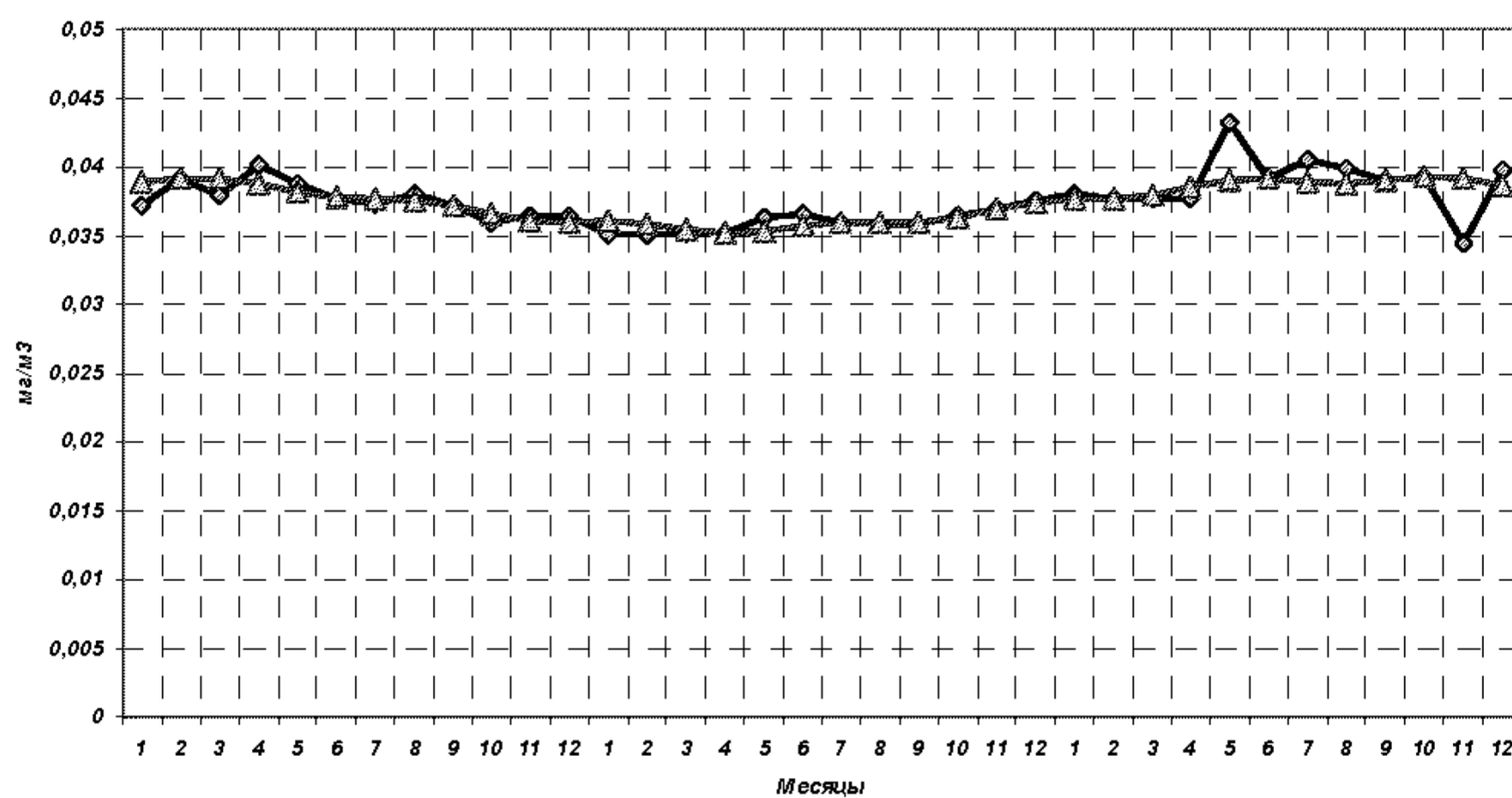
в) PM 2,5
