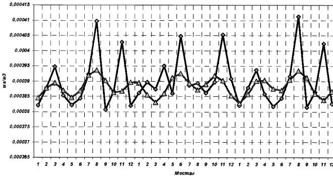
д) Cd
