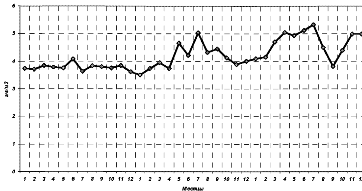
б) CO
