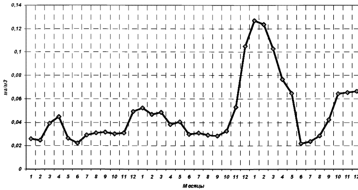
a) NO 2
