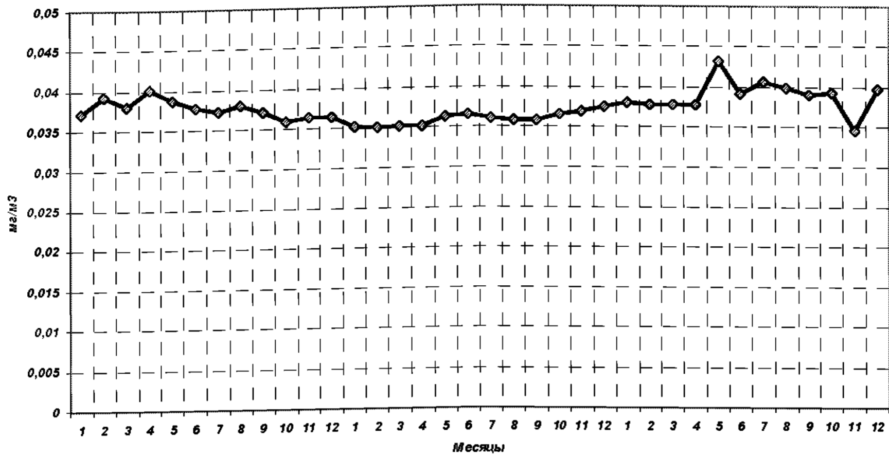
В) PM_{2,5}
