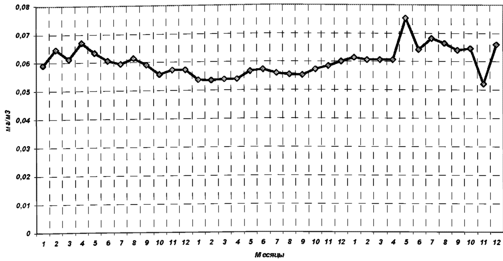
Г) PM_{10}
