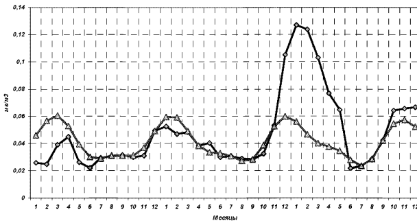
а) NO 2
