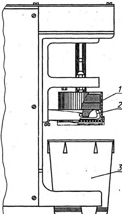
Рисунок 1 — Автоматический прибор для отделения клейковины
